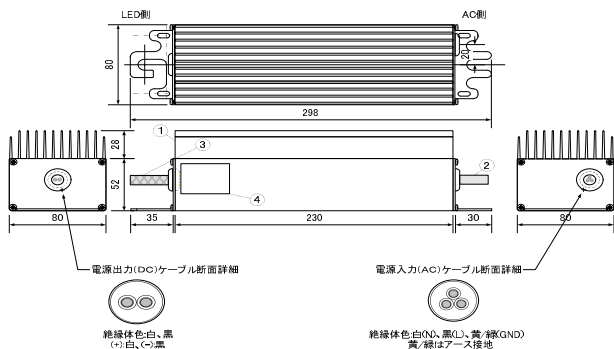
【電源外形図】
