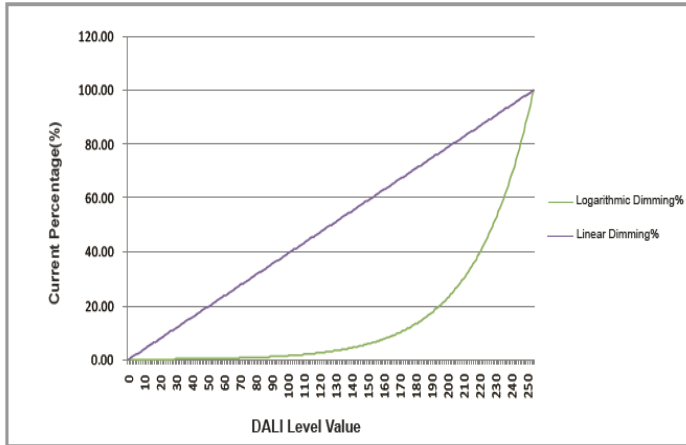
調光カーブ
