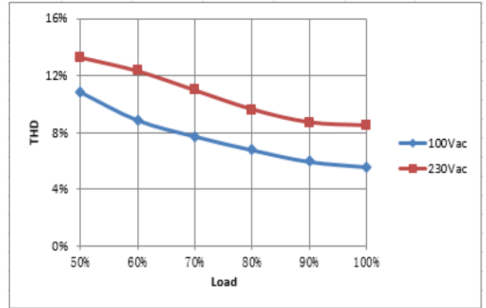
THD VS. 負荷曲線 (300mA for ref.)
