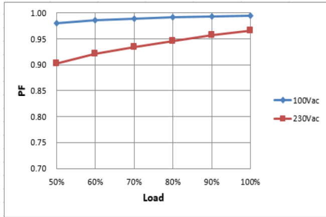
力率 VS. 負荷曲線 (300mA for ref.)
